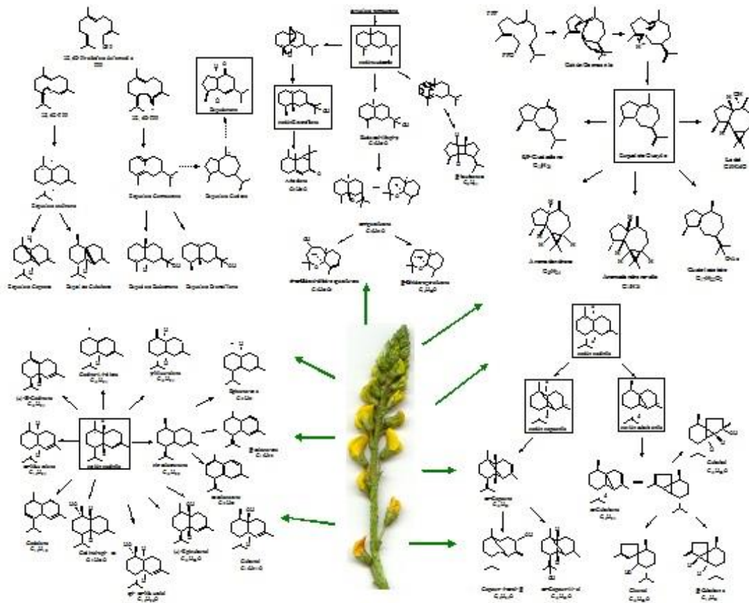
Fig. 2: Componentes principales del aceite esencial de A. boronioides (González, 2002)
