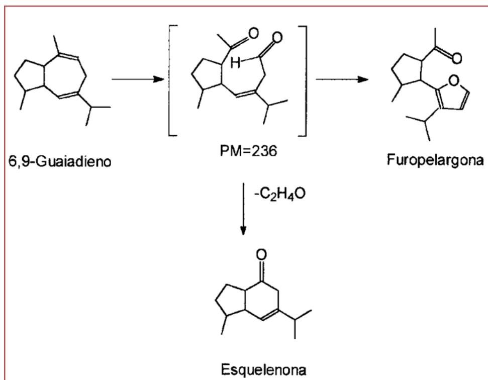
Fig 1. Biosíntesis propuesta para esquelenona
