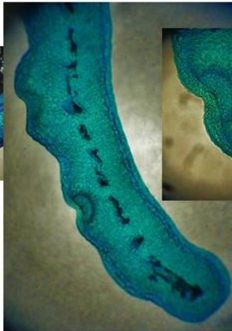
Estructura microscópica de las estructuras glandulares en tallos y hojas (40x).
